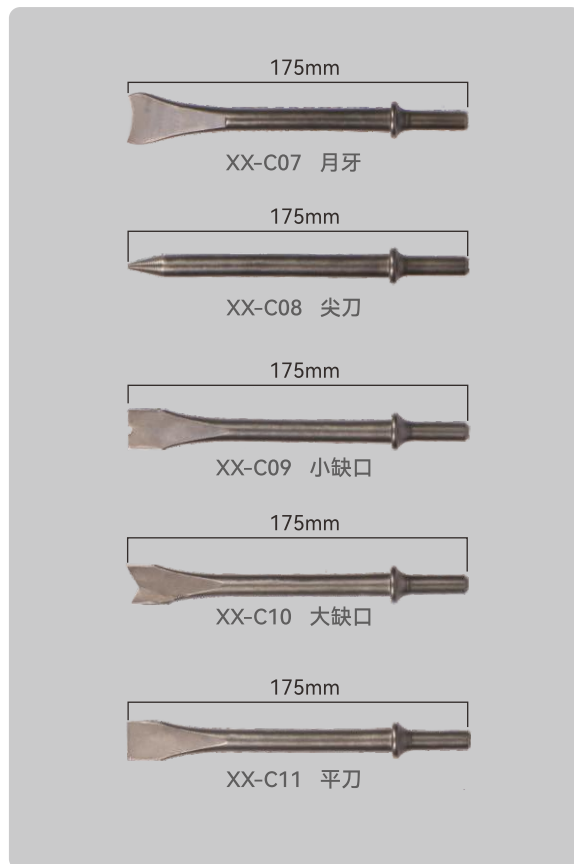
除锈针铲刀
